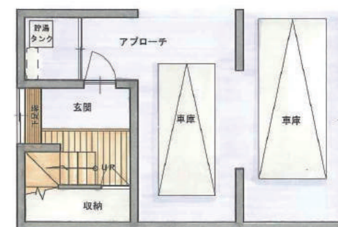
1階平面図
