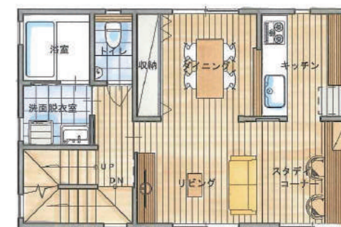
2階平面図
